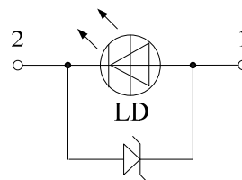
Zener Diode
